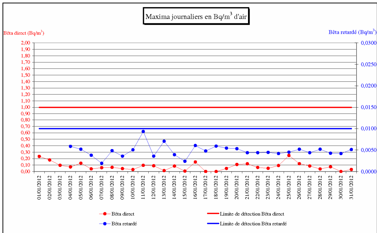
Bêta direct (temps t) - bêta retardé (temps t + 5j 10h) 4
