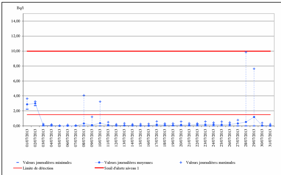
Evolution des activités volumiques de la voie « gamma total » - Juillet 2013
