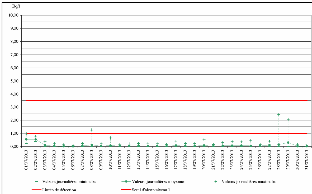
Evolution des activités volumiques de la voie « gamma [320 keV ; 400 keV] » - Juillet 2013
